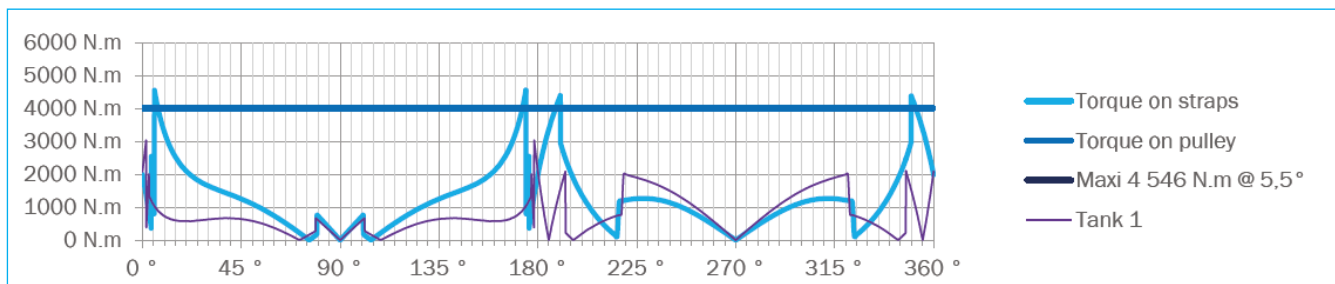
Figure 3 : Effet d'un déport de 10 cm du centre de gravité. En violet : CDG centré en bleu CDG déporté. Pour une masse identique, selon profil ci-dessus
