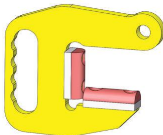
F crochets avec protection polyuréthane
